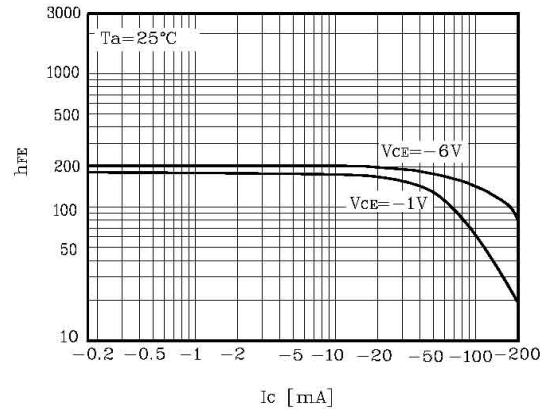
h_{FE}-I_C
